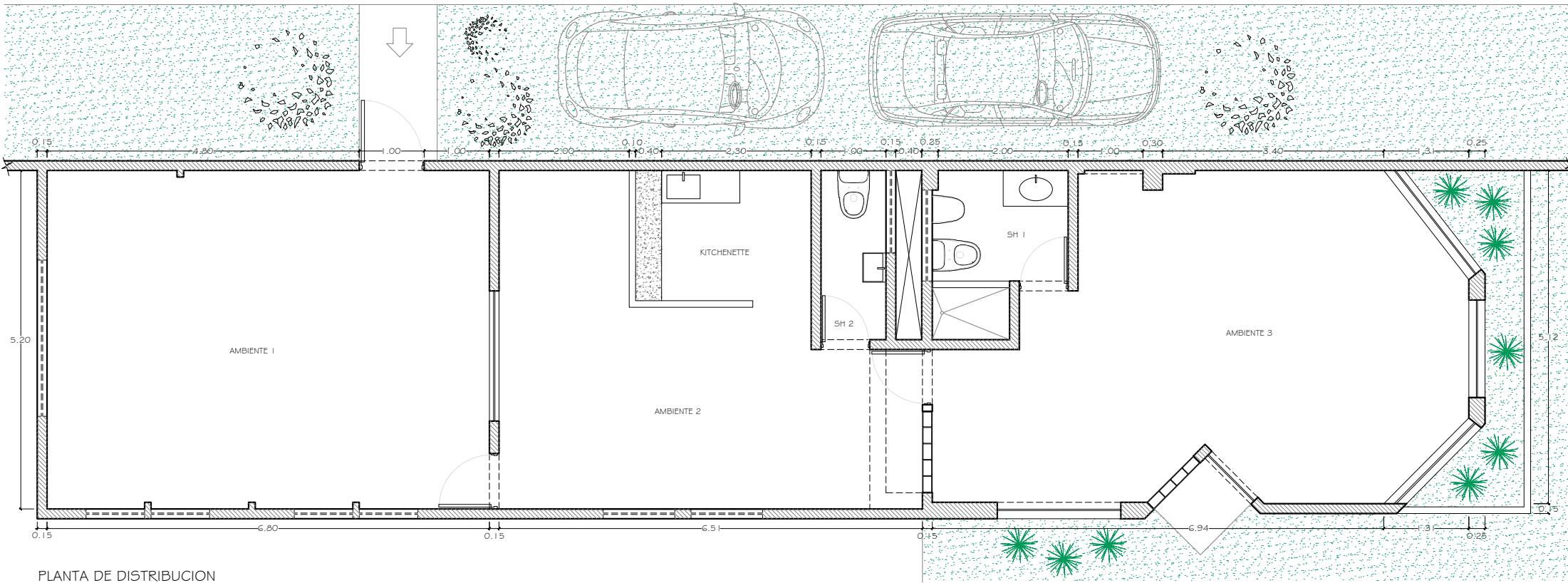
PLANTA DE DISTRIBUCION
